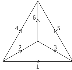
FIGURE 8 – Orientation de référence de K_4 . Ses circuits sont 1\bar{2}3 , 1\bar{4}5 , 2\bar{4}6 , 3\bar{5}6 , 13\bar{4}6 , 1\bar{2}5\bar{6} , 2\bar{3}45 , et leurs opposés. Ses cocircuits sont 124 , \bar{1}35 , 23\bar{6} , 456 , 12\bar{5}\bar{6} , \bar{1}\bar{3}46 , 2345 , et leurs opposés.
