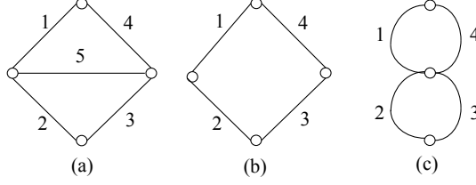
FIGURE 4 – (a) G ; (b) G \setminus 5 et (c) G/5 .
