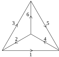
FIGURE 11 – Dual de K_4 (pour l'orientation de référence). Voir Figure 5 pour dualité des graphes planaires.
